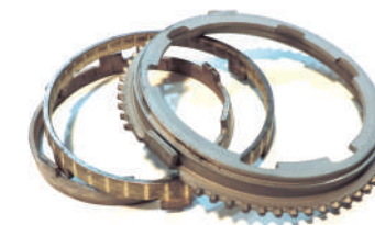
82000014N ENGRANAJE DE 2° z38 (38x17) y M/ATRÁS z27
