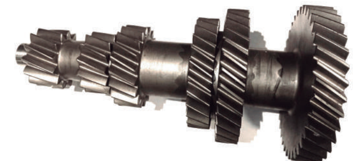
88002N QUINTUPLE z13-13-19-26-32-37
