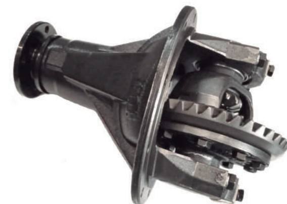
NM-215 /217 / 219 RELACIONES 11x41 - 9x41 - 9x43 28 ESTRIAS
