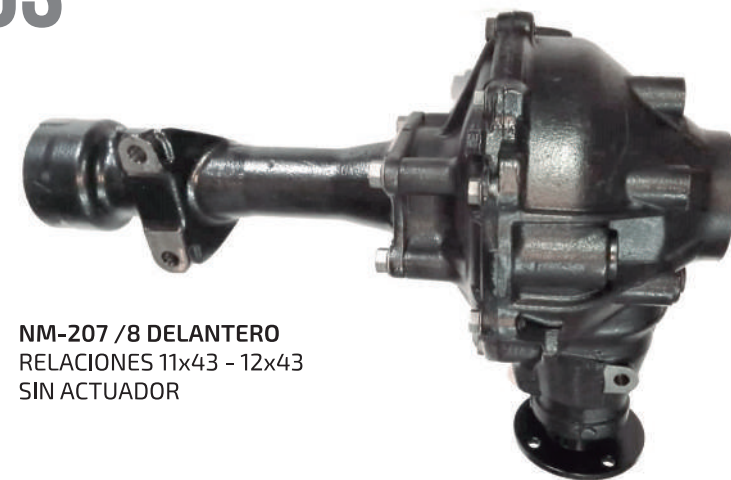
NM-200 /6 RELACIONES 9x41 - 10x41 - 11x41 - 11x43 - 12x43 COMUN Y AUTOBLOCANTES
